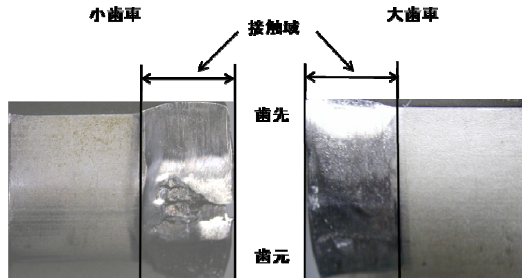
試験歯車 I-I(試験段階9)
