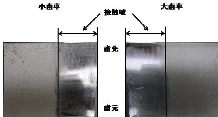
試験歯車 C-I(試験段階9)
